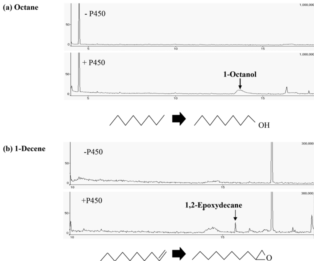
Fig. 4. GC-MS analysis.
